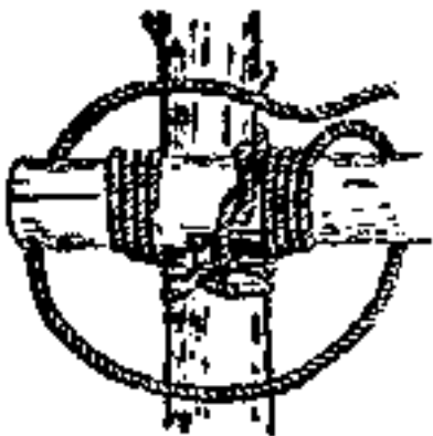
Amarre Cuadrado. Principiase con un ballestrinque. Háganse vueltas para atorar en ángulo recto con las vueltas principales. Terminese con el ballestrinque.
